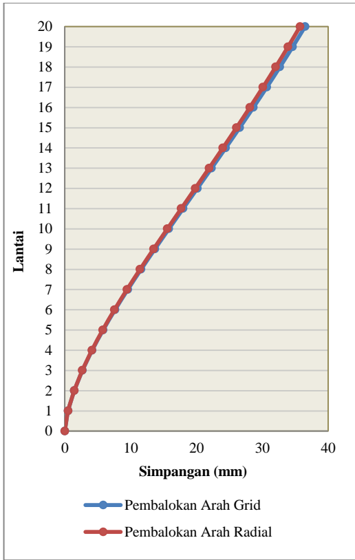
Grafik 2. Simpangan Maksimum akibat Gempa Dinamik untuk Kasus A
