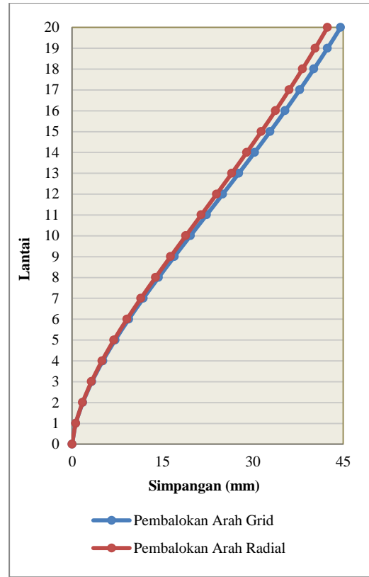
Grafik 3. Simpangan Maksimum akibat Gempa Statik untuk Kasus B
