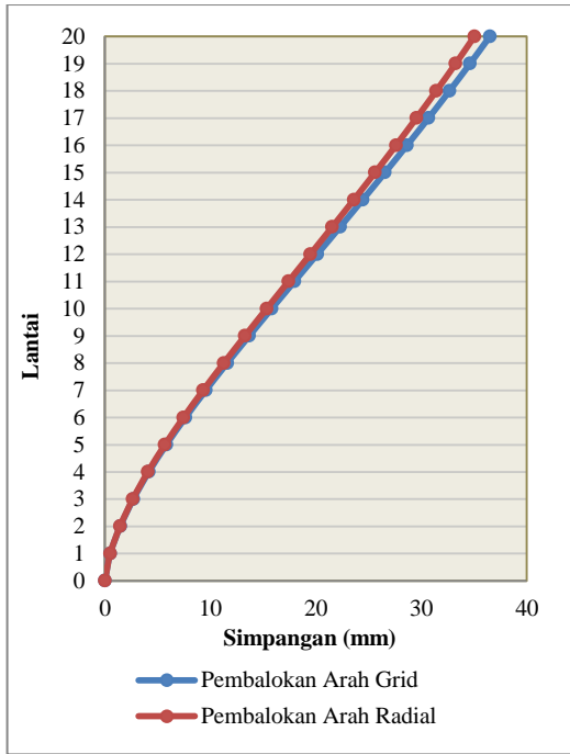
Grafik 4. Simpangan Maksimum akibat Gempa Dinamik untuk Kasus B
