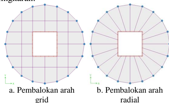
Gambar 1. Potongan Melintang Model Bangunan Dengan Bentuk Dasar Lingkaran
