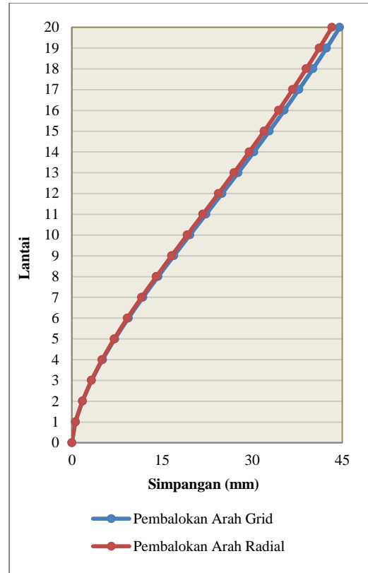
Grafik 1. Simpangan Maksimum akibat Gempa Statik untuk Kasus A
