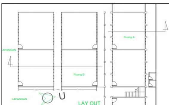
Gambar 2. Lay Out Sekolah Dasar Negeri 6 Manado Sumber: Dokumentasi Pribadi
