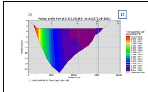
Gambar 7. Penampang DD saat spring-
