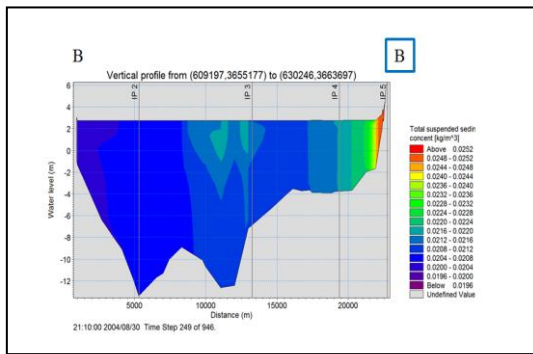
Gambar 5. Penampang BB saat spring
