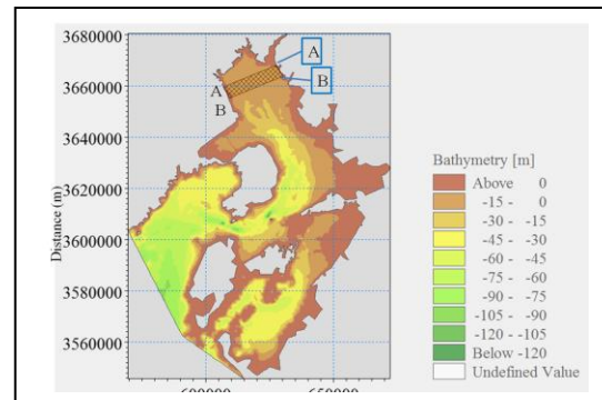
Gambar 2. Area AA-BB sebagai kontrol volume
