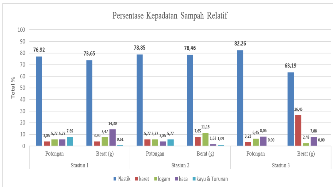
Gambar 3. Persentase kepadatan sampah anorganik relatif tiap stasiun
