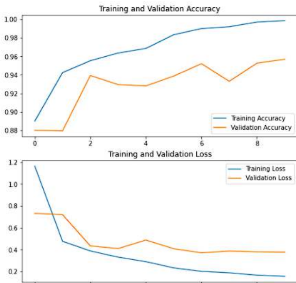
Gambar 8. Grafik Perbandingan Hasil Latih dan Validasi Model C
