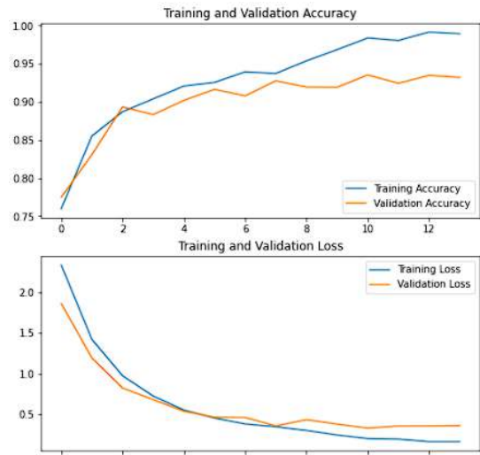
Gambar 7. Grafik Perbandingan Hasil Latih dan Validasi Model B
