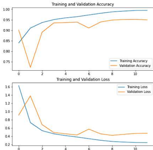
Gambar 6. Grafik Perbandingan Hasil Latih dan Validasi Model A
