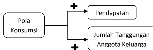
Gambar 2. Kerangka Konseptual
