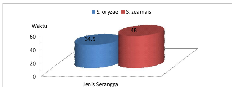
Gambar 4. Diagram Batang Siklus Hidup Sitophilus oryzae dan Sitophilus zeamais Pada Beras dan Jagung Pipilan Di Laboratorium
