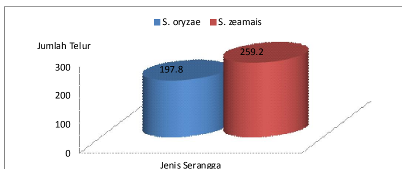
Gambar 6. Diagram Batang Fekunditas Sitophilus oryzae dan Sitophilus zeamais pada Beras dan Jagung Pipilan Di Laboratorium.
