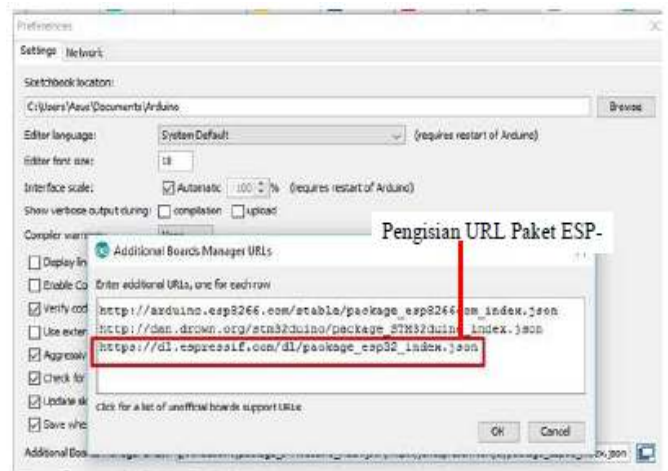
Gambar 14. Proses memasukkan package ESP32
