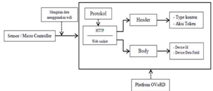
Gambar 8. Diagram blok pengiriman data pada platform ovord
