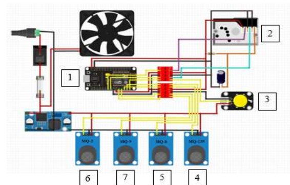
Gambar 10. Desain dan rangkaian komponen
