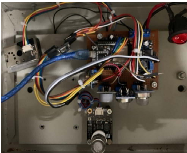
Gambar 12. Implementasi perangkat keras
