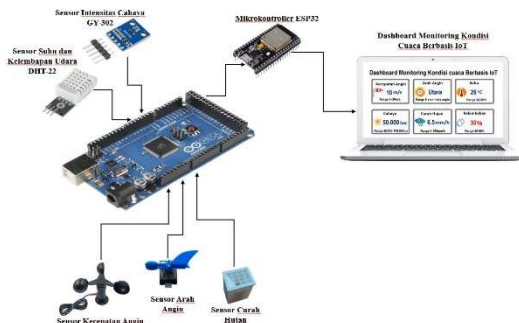
Gambar 3. Desain Komponen
