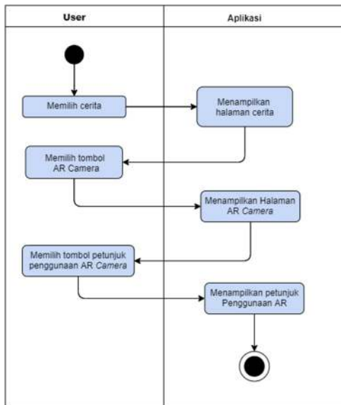
Gambar 5. Activity Diagram Petunjuk penggunaan AR camera
