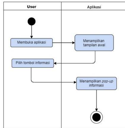
Gambar 7. Pop-up informasi aplikasi
