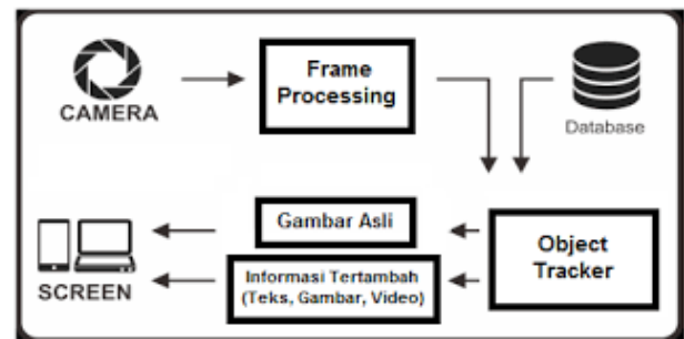
Gambar 1. Prinsip kerja Vuforia
