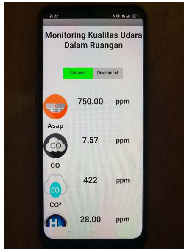
Gambar 20. Tampilan Sistem Monitoring Kualitas Udara
