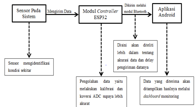
Gambar 9. Bagan Sistem Monitoring Kualitas Udara
