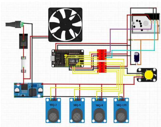
Gambar 11. Desain dan Rangkaian Komponen
