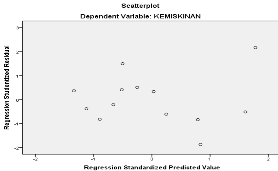
Gambar 1 Uji Heterokedastisitas
