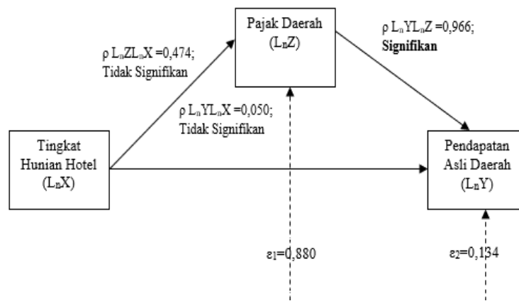
Gambar 5. Hasil Uji Hipotesis Analisis Jalur
