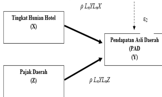
Gambar 4. Model persamaan sub-struktural 2
