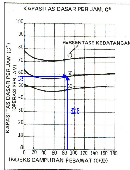
Grafik 1. Hasil Kapasitas Dasar (Kd), kondisi IFR
