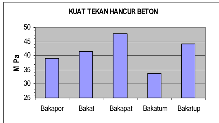
Grafik 11: Hubungan Jenis Beton dan Kuat Tekan Hancur
