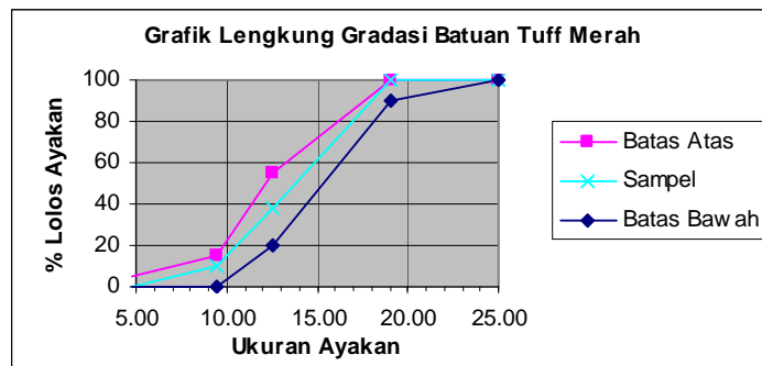
Grafik 4: Hubungan Ukuran Ayakan dengan Persentase Lolos Batuan Tuff Merah
