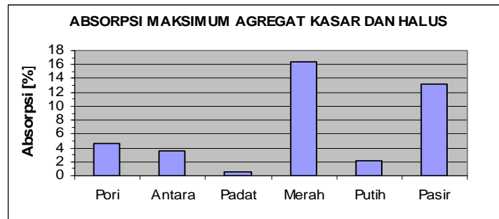
Grafik 8: Hubungan Jenis Agregat dan Absorpsi Maksimum
