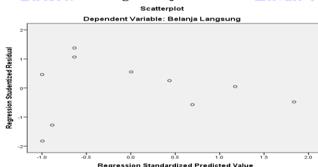
Gambar 3. Diagram Uji Heterokedastisitas
