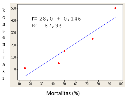
Gambar 8. Grafik Analisis regresi Halimeda sp hubungan moratlitas dan konsentrasi
