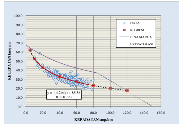
Gambar 11. Hubungan antara Kecepatan dan Kepadatan
