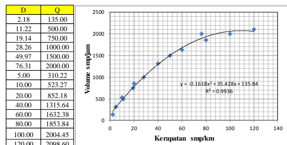
Gambar 13. Kurva Hubungan antara Kepadatan dan Volume
