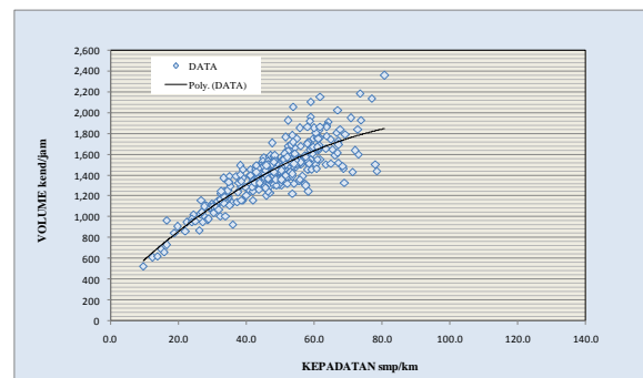
Gambar 12. Hubungan antara Kepadatan dan Volume
