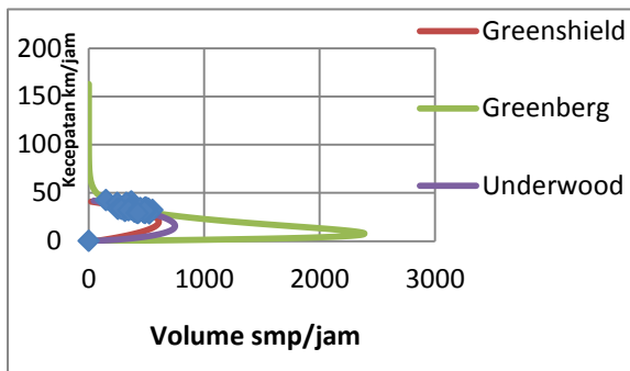
Gambar 9. Kurva Hubungan Matematis antara Volume-kepadatan model Greenshield, Greenberg dan Underwod untuk hari senin
