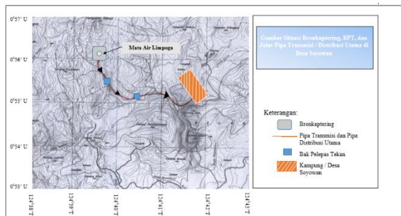
Gambar 3. Gambar Situasi Bronkaptering, BPT, Jalur Pipa Transmisi / Distribusi Utama Desa Soyowan
