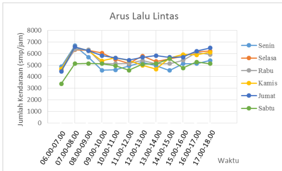
Gambar 2. Hubungan Total Kendaraan Setiap Jam
