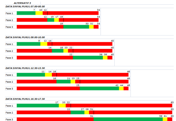
Gambar 4.8 Urutan Fase Sinyal Alternatif 3
