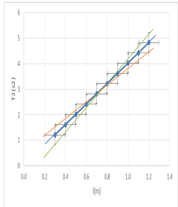
Gambar 2. Plot hubungan antara periode getaran dengan panjang tali bandul.
