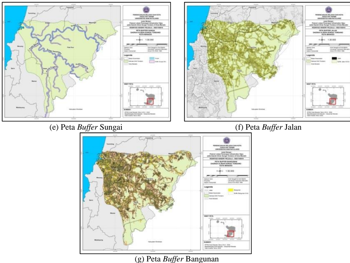
Gambar 2. Peta Karakteristik DAS Tondano berdasarkan faktor penentuan lokasi infrastruktur hijau (Penulis, 2022)
