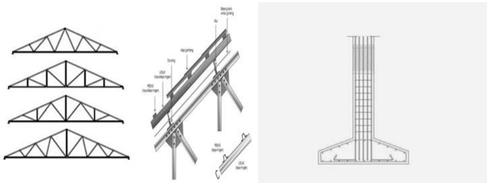
Gambar 6 : Struktur Rangka Baja Ringan dan Pondasi Telapak Sumber : Penulis 2017
