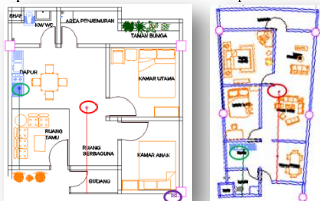
Gambar 13. Instalasi listrik tipe 42 (kiri) dan instalasi listrik tipe 84 (kanan) Sumber: Penulis, 2017
