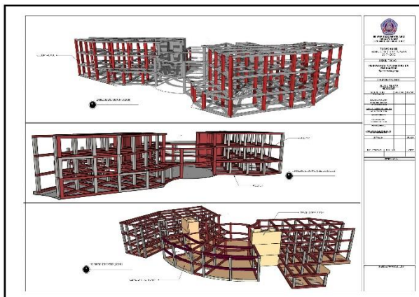
Gambar Isometri Struktur Gambar Potongan bangunan
