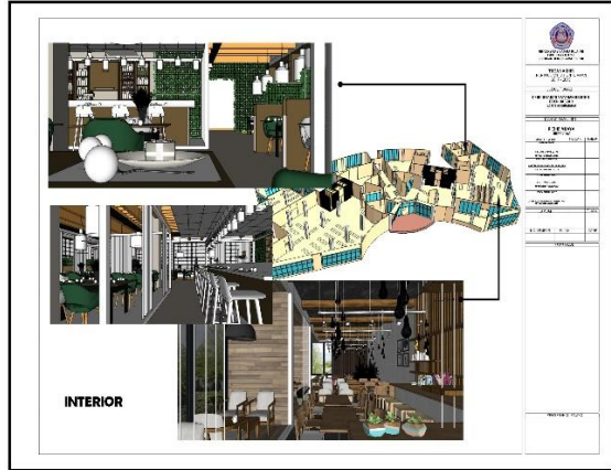
Konsep interior di buat agar pengguna merasa nyaman dengan penggunaan material kayu dan wallpaper bertekstur kayu, interior di buat dengan konsep natural agar pengguna juga merasa tenang saat bersosialisasi maupun membaca
