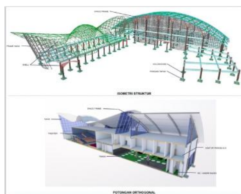
Gambar 21. Isometri Struktur dan Potongan Orthogonal
