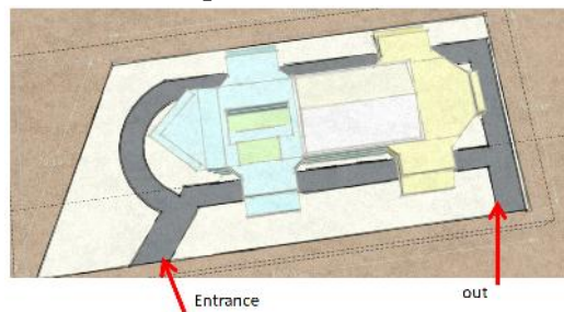
Gambar 6 Konsep Entrance dan Sirkulasi Tapak
