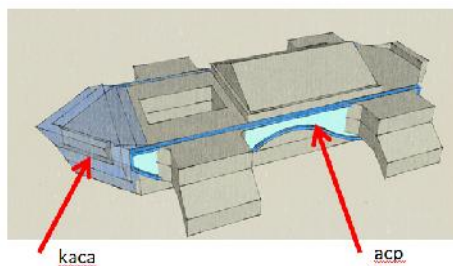
Gambar 8 Konsep Selubung Bangunan
