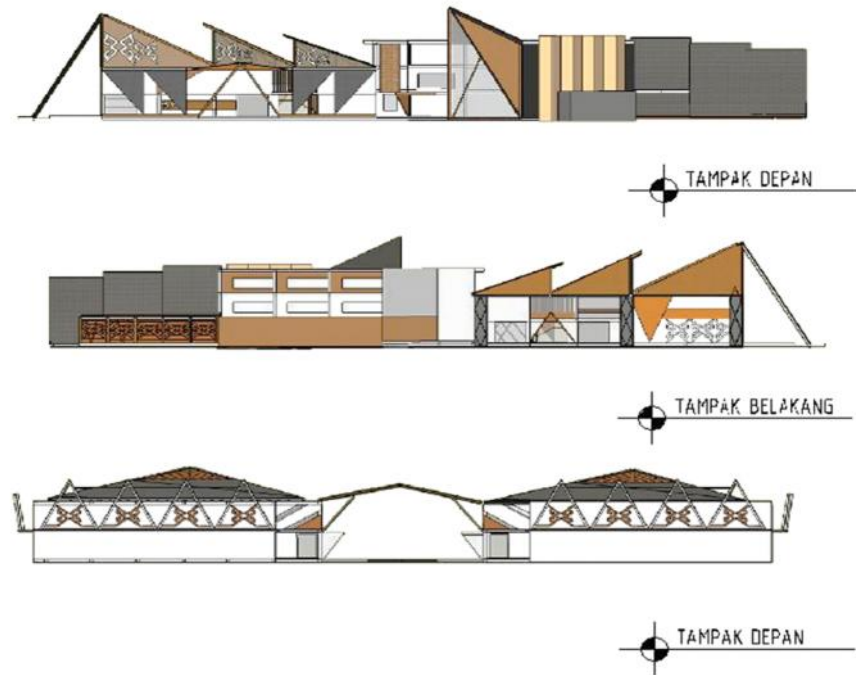
Gambar 6. Tampak Bangunan
