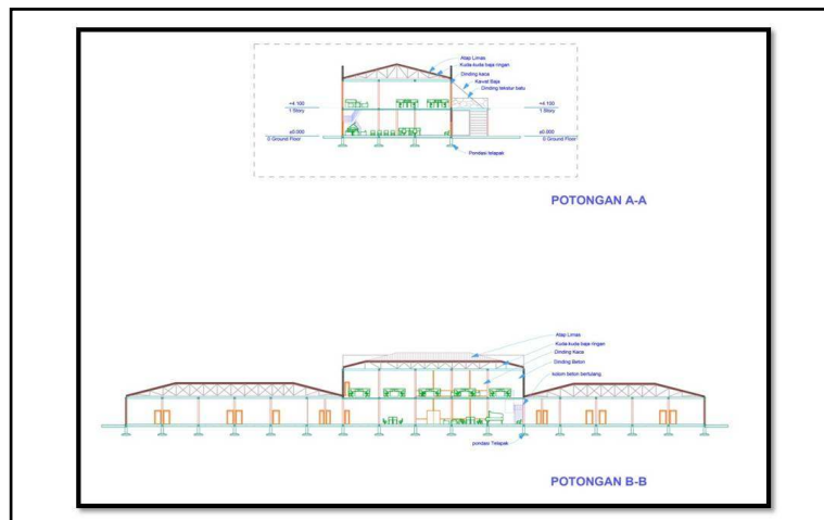
Gambar 14. Potongan Bangunan
