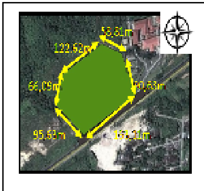
Gambar 3. Dimensi Tapak
