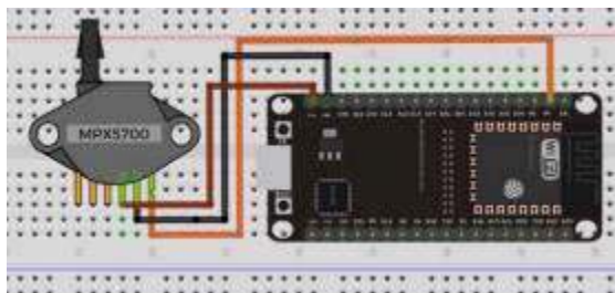
Gambar 5 Rangkaian Sensor MPX5700 dengan Mikrokontroler ESP32
