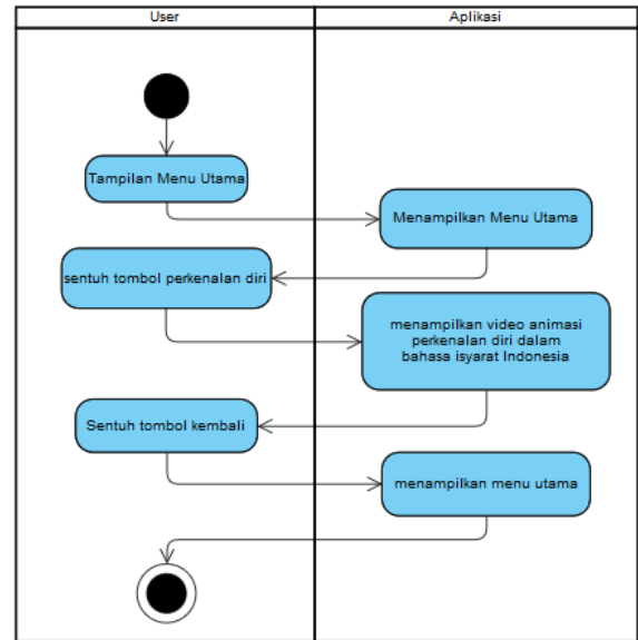
Gambar 3. Activity Diagram Menu Perkenalan Diri
