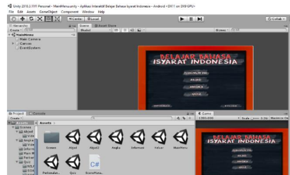
Gambar 11. Pembuatan Aplikasi
