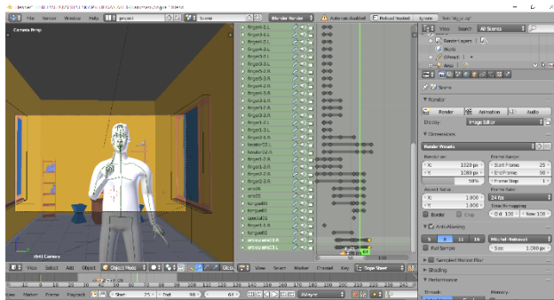
Gambar 10. Pembuatan Animasi
