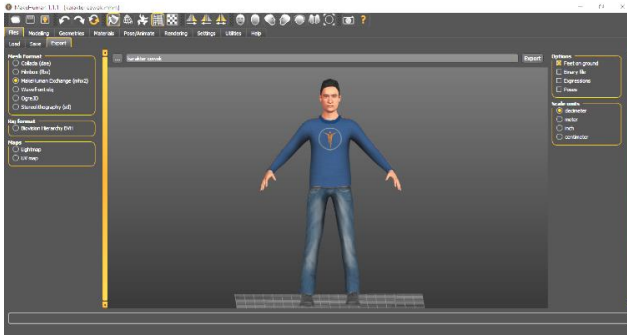
Gambar 8. Modeling Karakter
