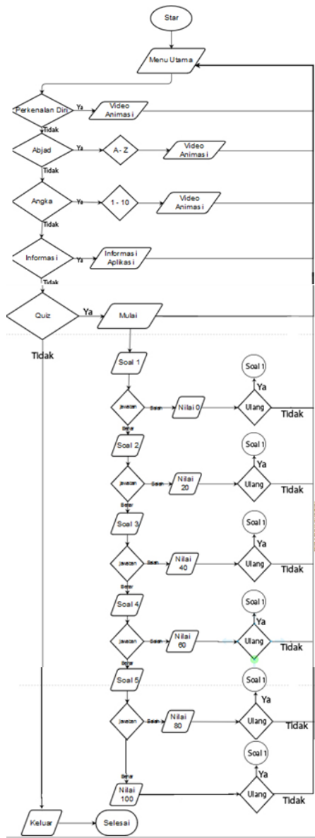
Gambar 1. Flowchart Aplikasi
