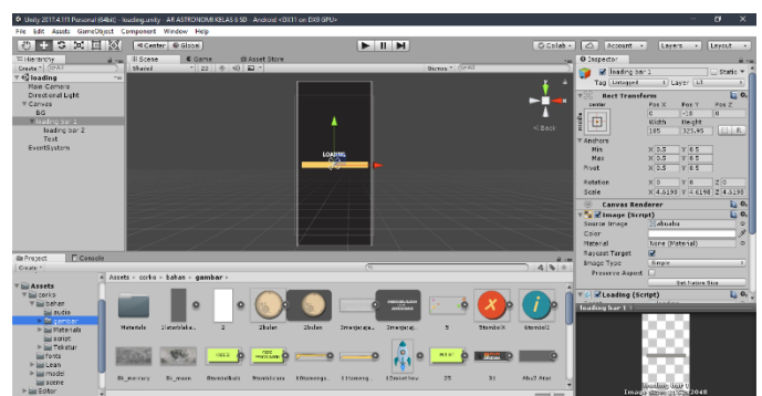
Gambar 14. Pembuatan Tampilan Splash Screen
