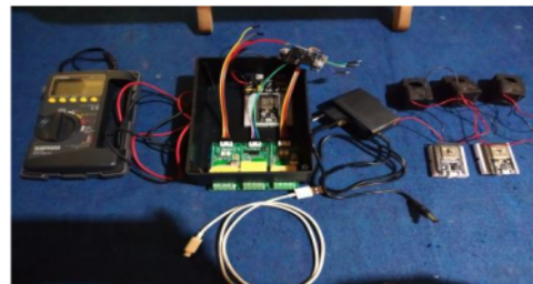
Gambar 6. Komposisi hardware sistem monitoring besaran listrik
