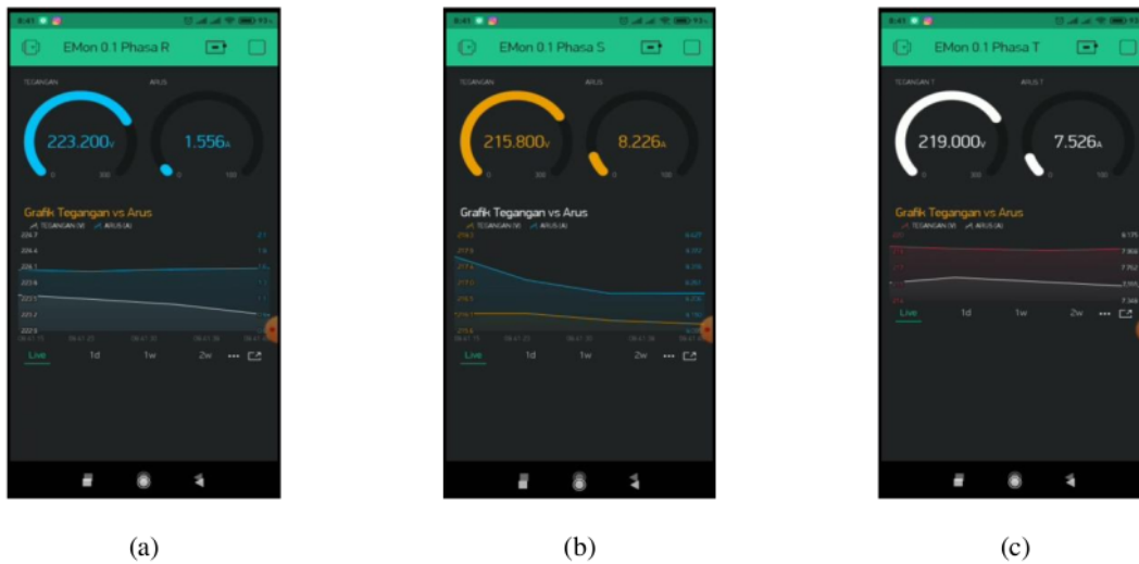
Gambar 8. Tampilan aplikasi monitoring besaran listrik pada smartphone (a) nilai besaran listrik pada phasa R (b) nilai besaran listrik pada phasa S dan (c) nilai besaran listrik pada phasa T.
