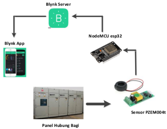
Gambar 5. Blok Diagram Sistem
