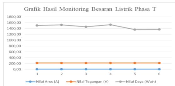
Gambar 12. Grafik Hasil Monitoring Besaran Listrik Fase T
