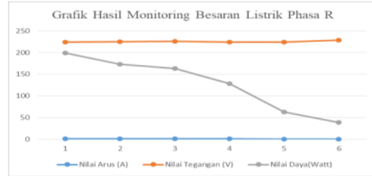
Gambar 10. Grafik Hasil Monitoring Besaran Listrik Fasa R
