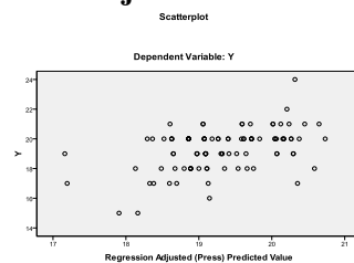
Gambar 2. Uji Heteroskedastisitas
