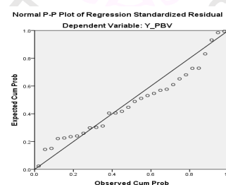
Gambar 3. Uji Normalitas
