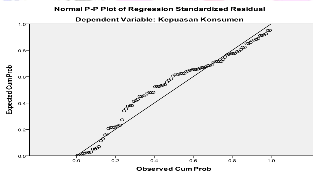
Gambar 2. Uji Normalitas
