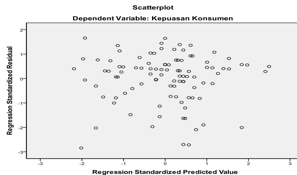
Gambar 3. Uji Heterokedastisitas
