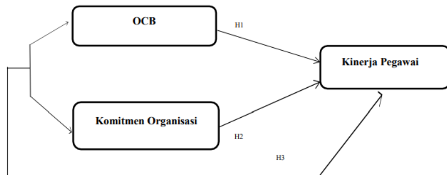
Gambar 1. Kerangka Berpikir
