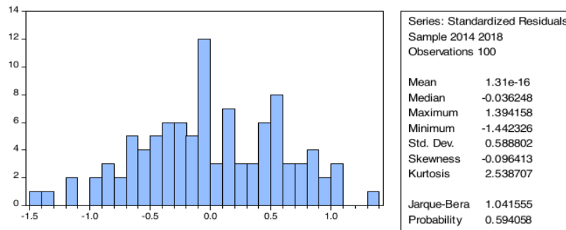
Gambar 1. Uji normalitas
