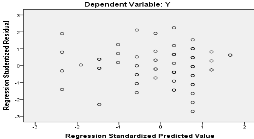
Gambar 4.2 Hasil Uji Heterokedastisitas Scatterplot
