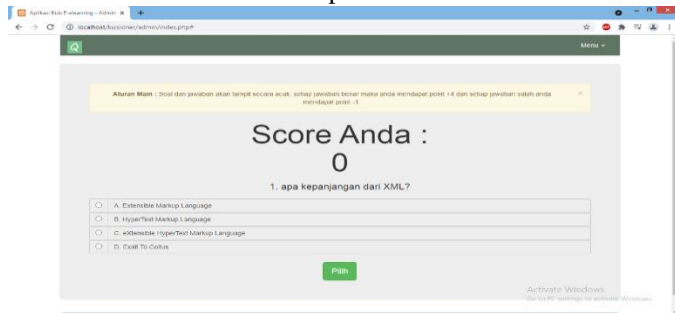
Gambar 21 Tampilan Kuis
