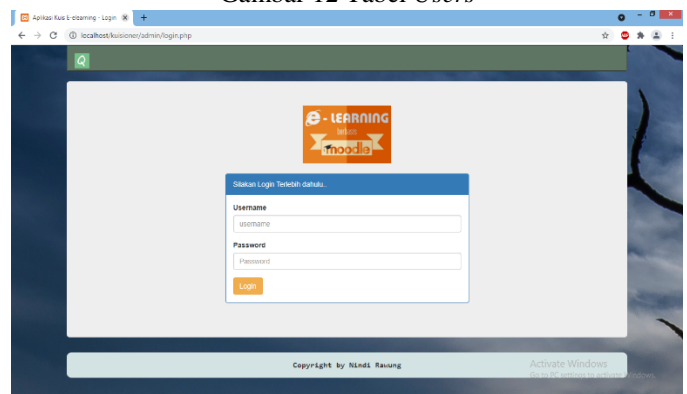
Gambar 13 Tampilan Login
