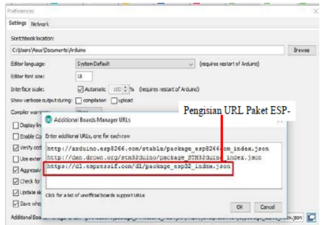
Gambar 12. Proses memasukkan package ESP32
