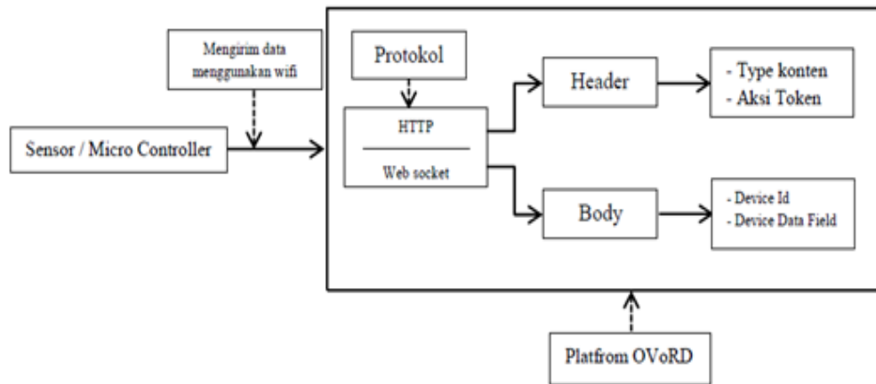
Gambar 6. Diagram blok pengiriman data pada platform ovord
