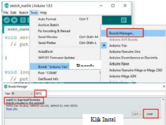
Gambar 13. Instalasi ESP32
