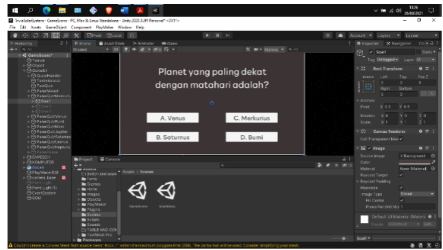
Gambar 28. Pembuatan Pertanyaan
