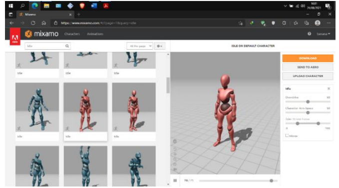
Gambar 21. Pembuatan Animasi
