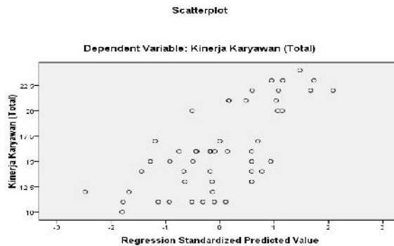
Gambar 3. Metode Grafik Scatterplot
