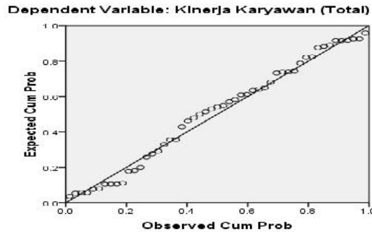
Gambar 2. Metode P-Plot Regression
