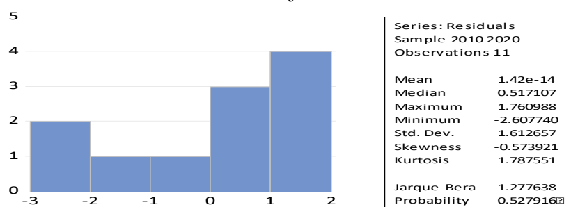
Gambar 2 Uji Normalitas
