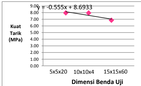
Grafik hubungan dimensi benda uji dan kuat tarik beton mutu tinggi pada umur beton 7 hari
