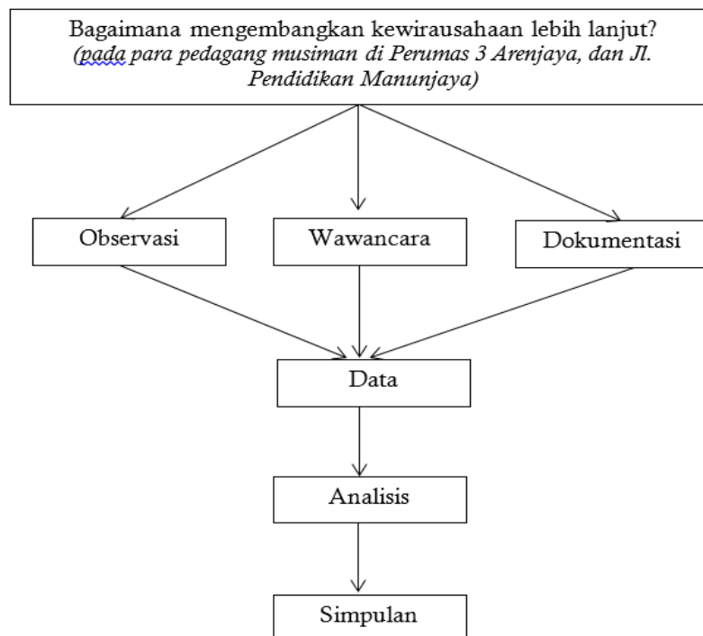
Gambar 3.2. Skema Rumusan Masalah
