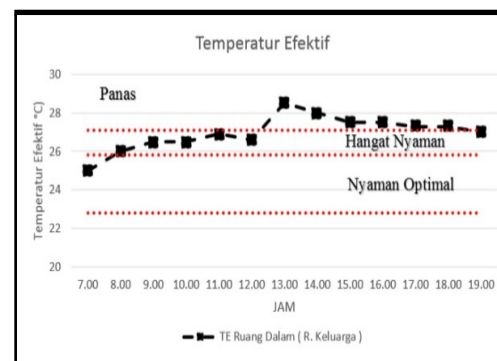
Gambar 6 Gambar Grafik Temperatur Efektif Pada Rumah Panggung
