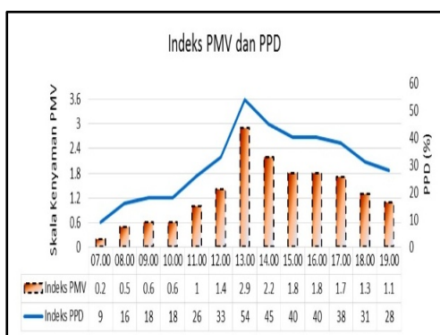
Gambar 7 Gambar Perhitungan Indeks PMV dan PPD Pada Rumah Panggung
