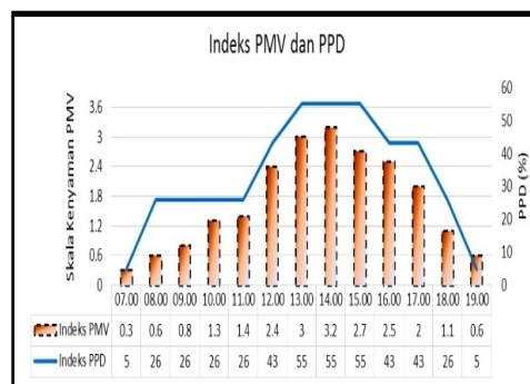
Gambar 5 Gambar Perhitungan Indeks PMV dan PPD Pada Rumah Lanting
