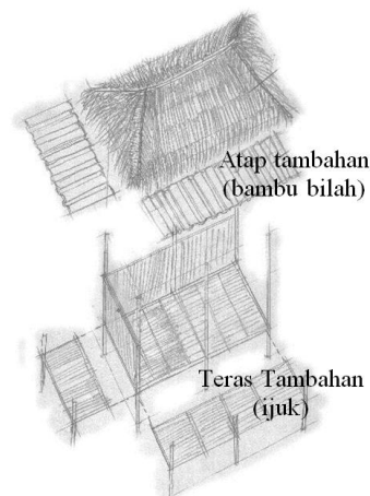
Gambar 6 Isometri beruqaq Agung Perumbak Sumber: Sketsa pribadi
